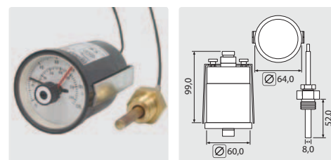
1/2" M. Contact 5 A - 250 V (AC1). Indication de température 0 - 120 °C
